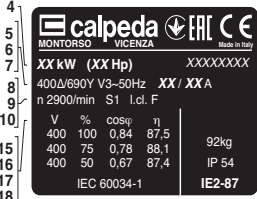
电机牌图示
