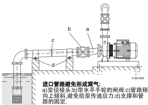
图2 管路连接
